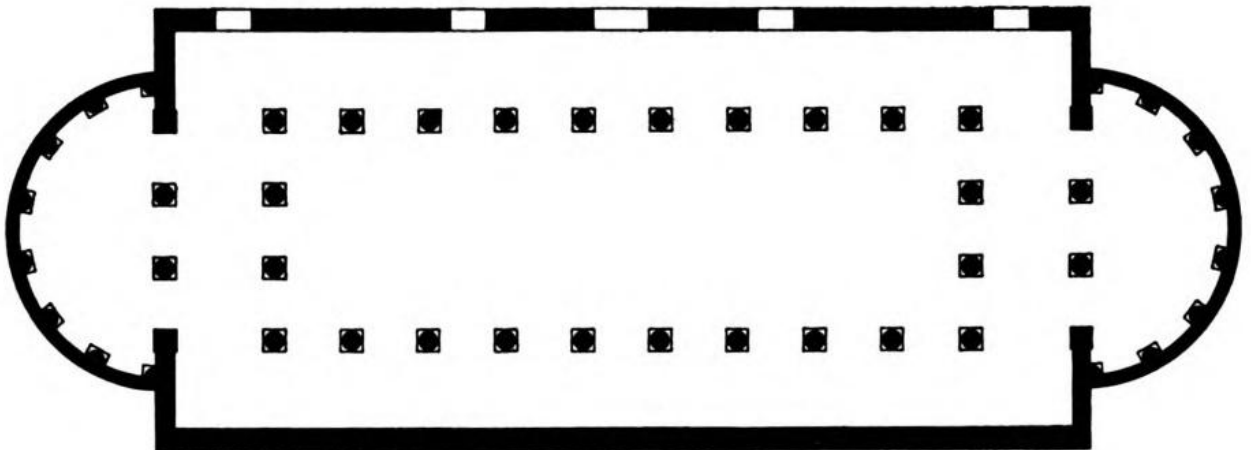
ichnographia basilicae Augustae Rauracorum prope Basileam sitae
